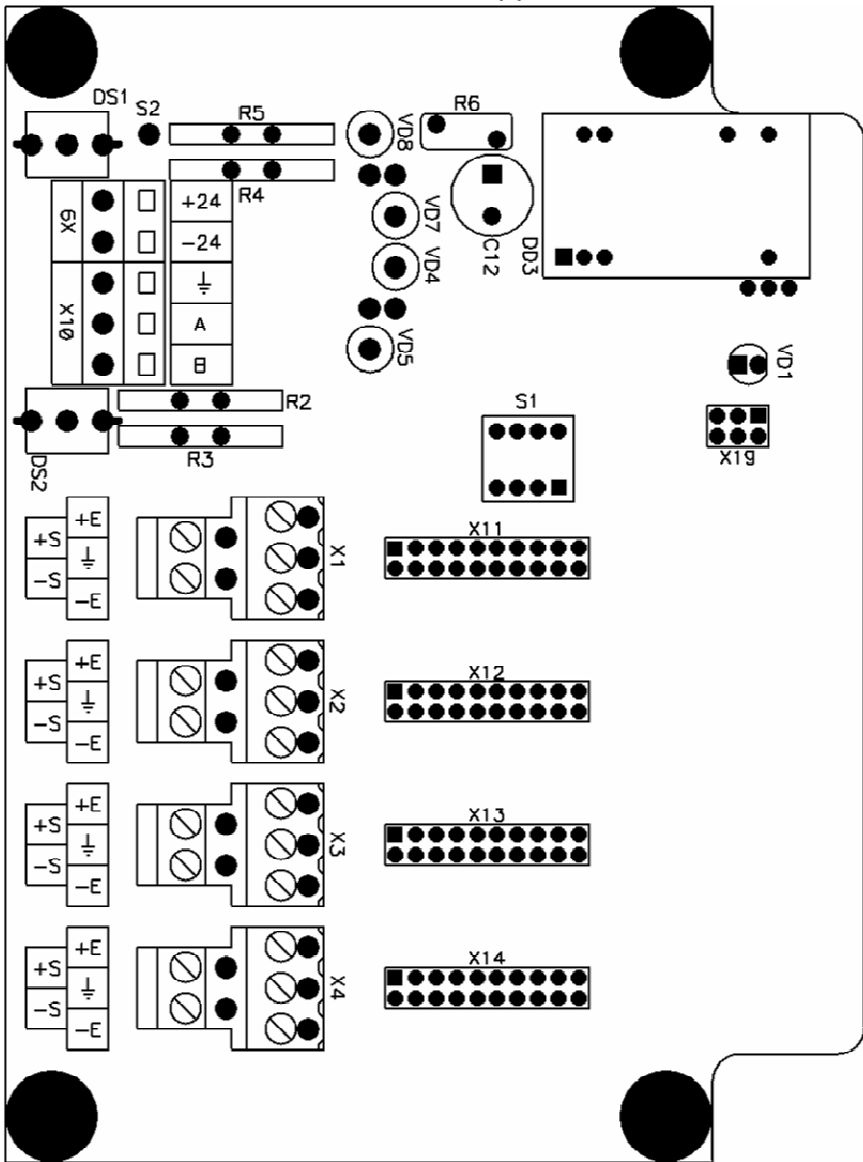
Приложение 1 Рис.1 Плата ПД-004
